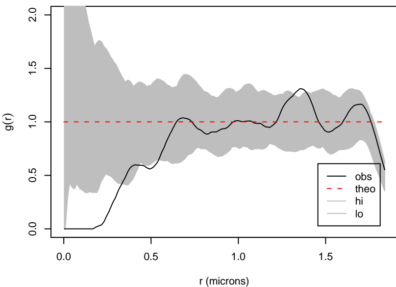
Cell 1 myofibrils PCF (Poisson envelopes)
